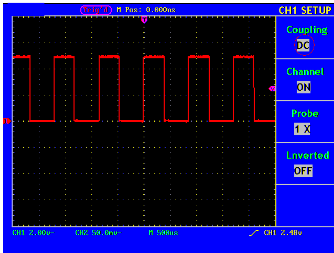
Fig. 16 DC Coupling
